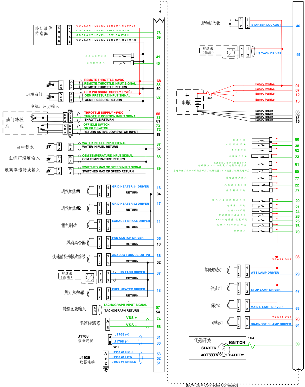
Figure 4-2: ISB4/ISB e 接线图 (OEM 接线口 B)
