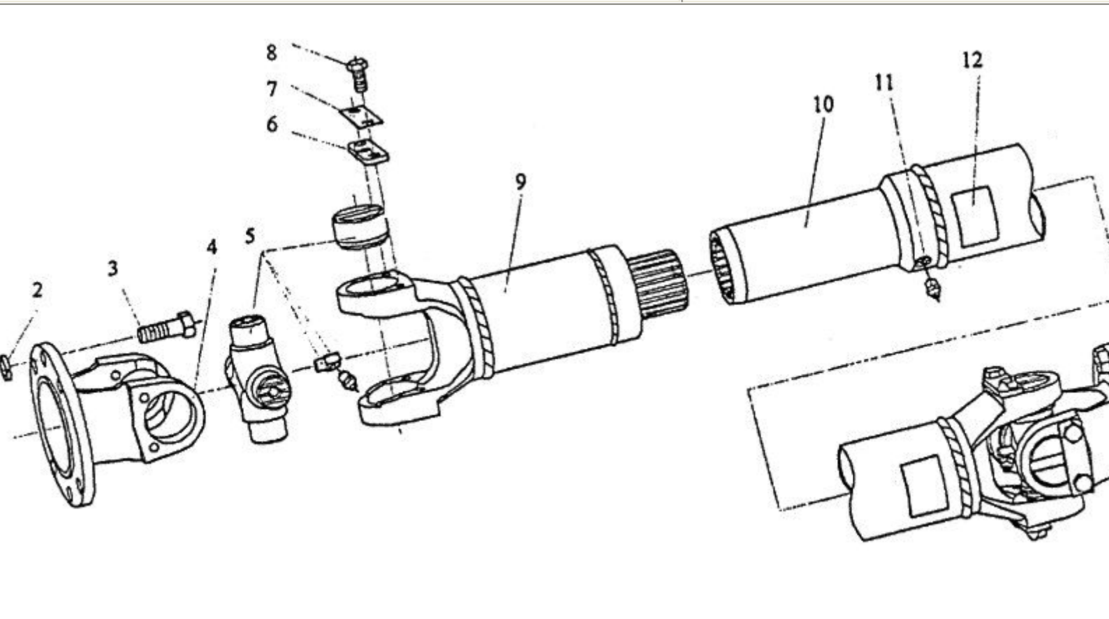
传动轴
