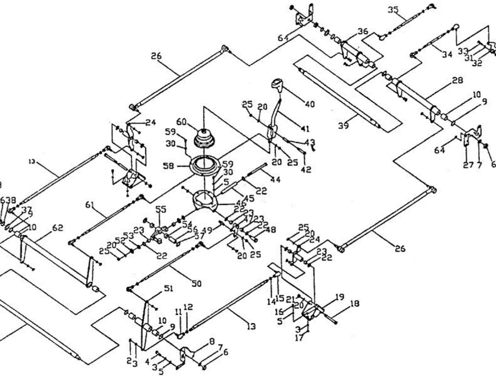
变速操纵机构
