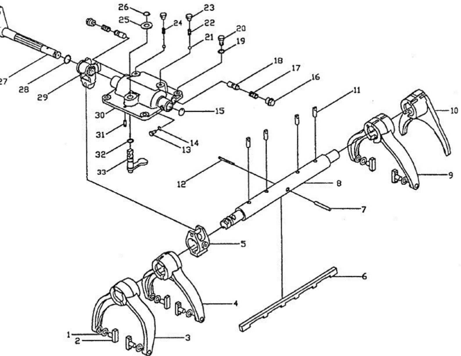
变速器顶盖及换档机构
