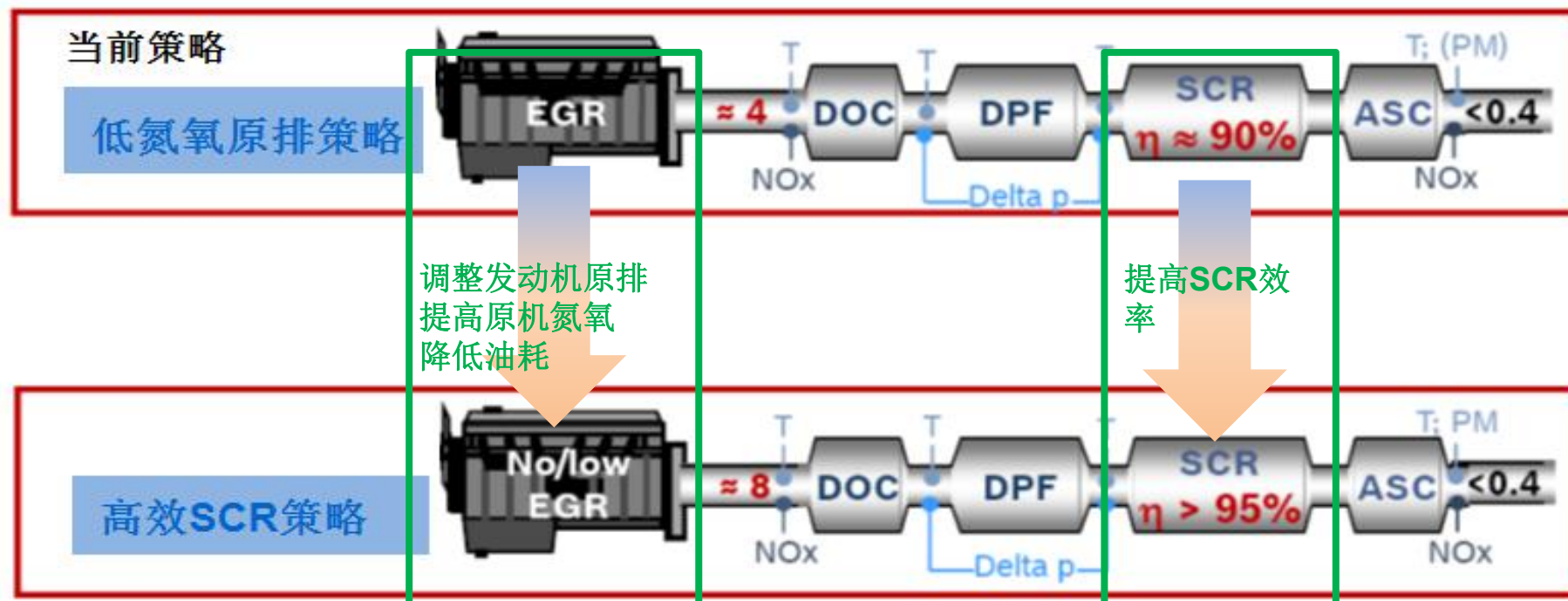
国六技术路线图
